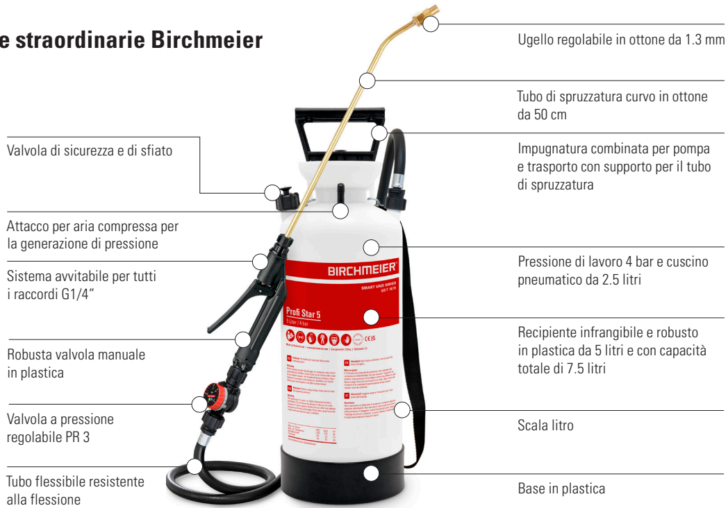
Profi Star 5 N. art. 11663301
